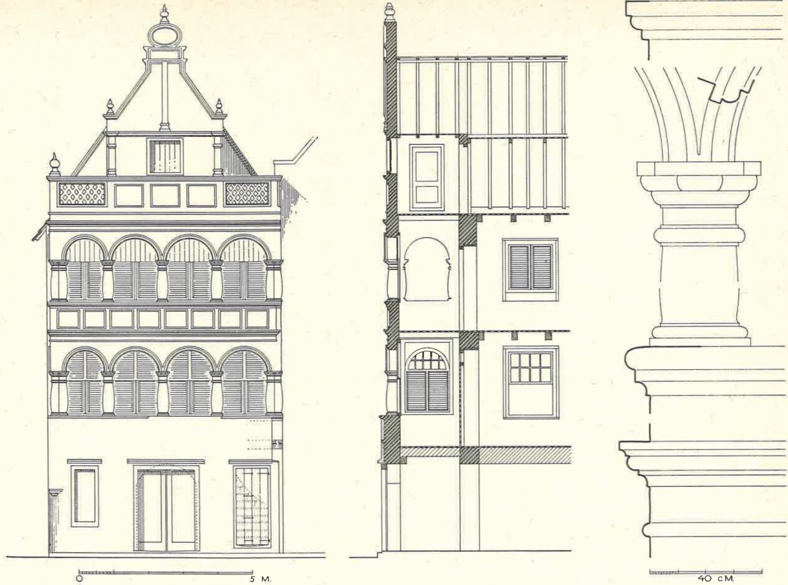
Fig. 29. Herenstraat 35. Voorgevel, lengtedoorsnede en geveldetails
